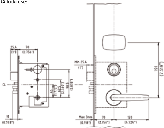
ANSI DA lockcase:
